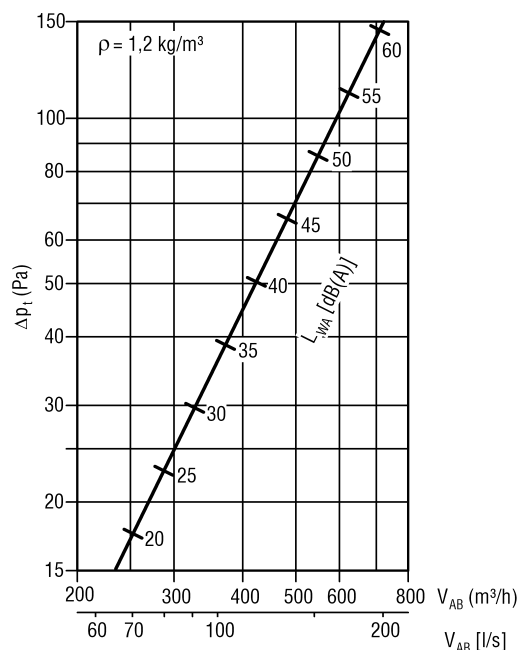
FLAQ-...-310-... with SK-Q-19-A-...
