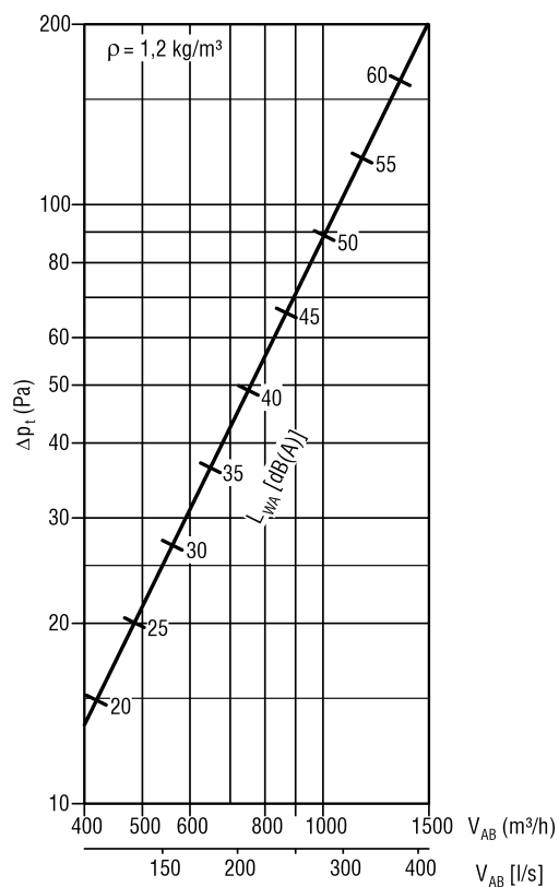
FLAQ-...-400-... with SK-Q-19-A-...
