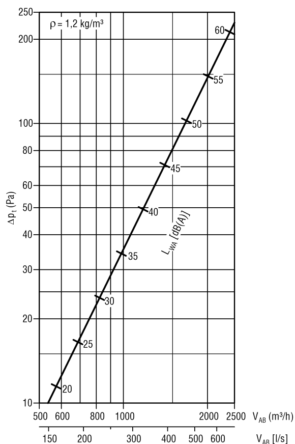
FLAQ-...-500-... with SK-Q-19-A-...
